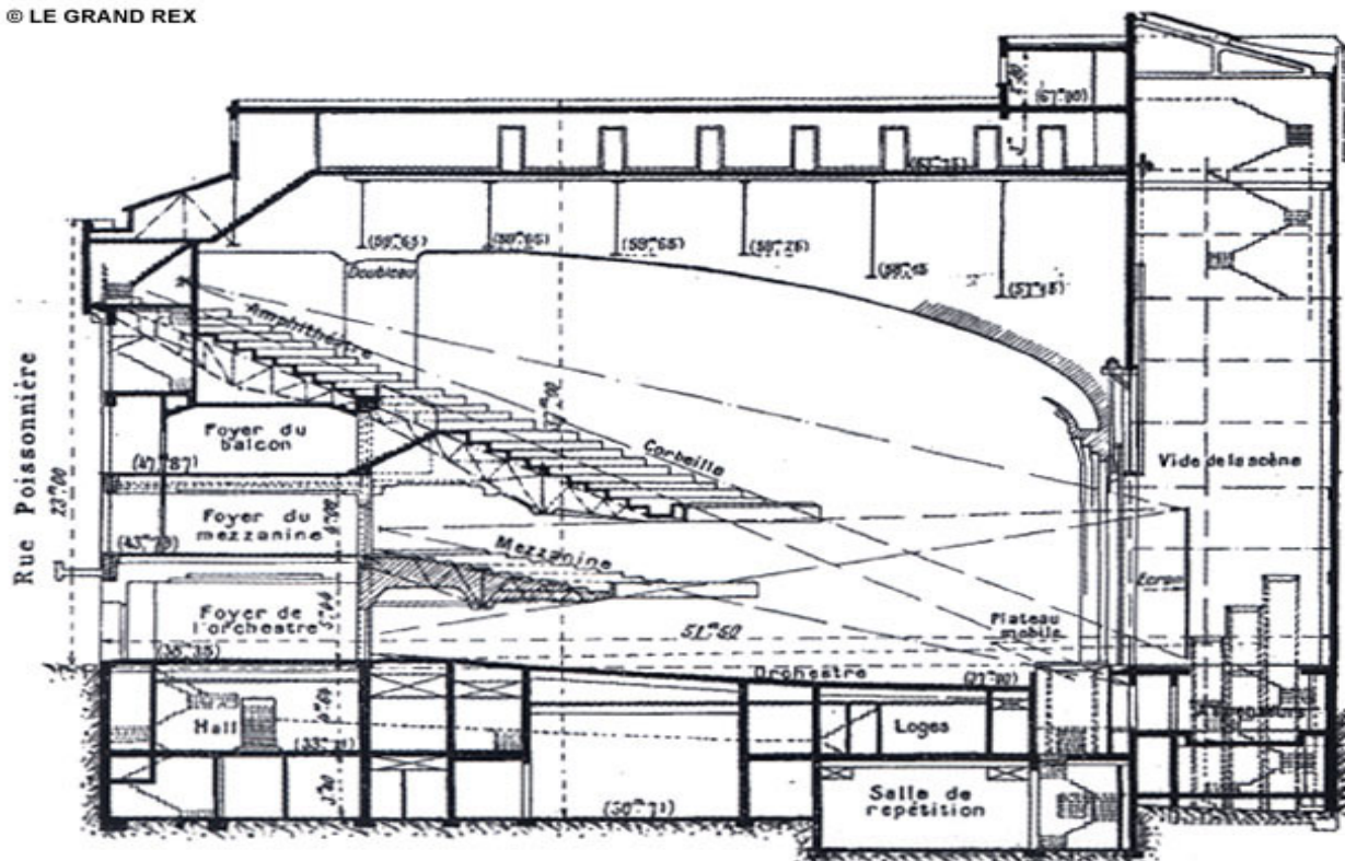
Slika 1 – Presek bioskopske sale "Le Grand Rex" - Pariz
